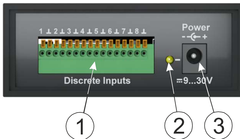
Рисунок 2 – Внешний вид задней панели адаптера iNode-Sense
