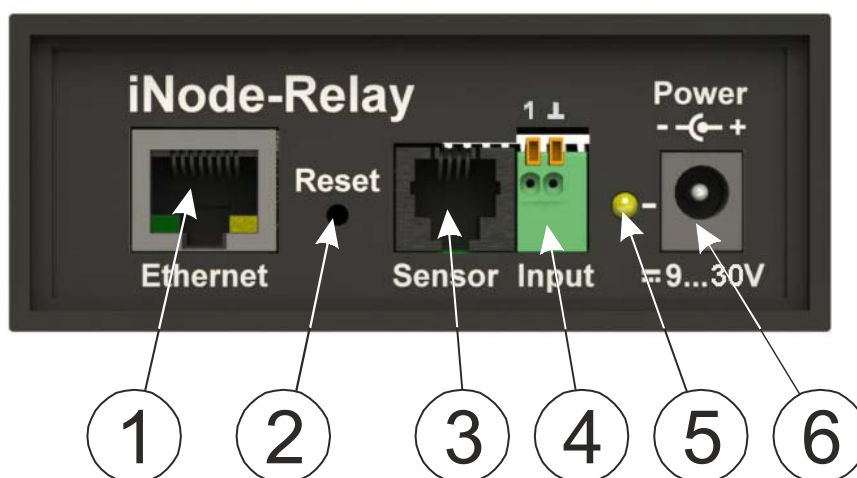
Рисунок 3 – Внешний вид передней панели адаптера iNode-Relay
