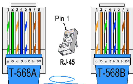
Рисунок 5 – Схема электрическая сетевого кабеля Ethernet 100Base-TX/10Base
