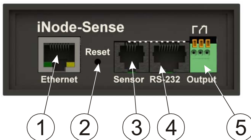
Рисунок 1 – Внешний вид передней панели адаптера iNode-Sense
