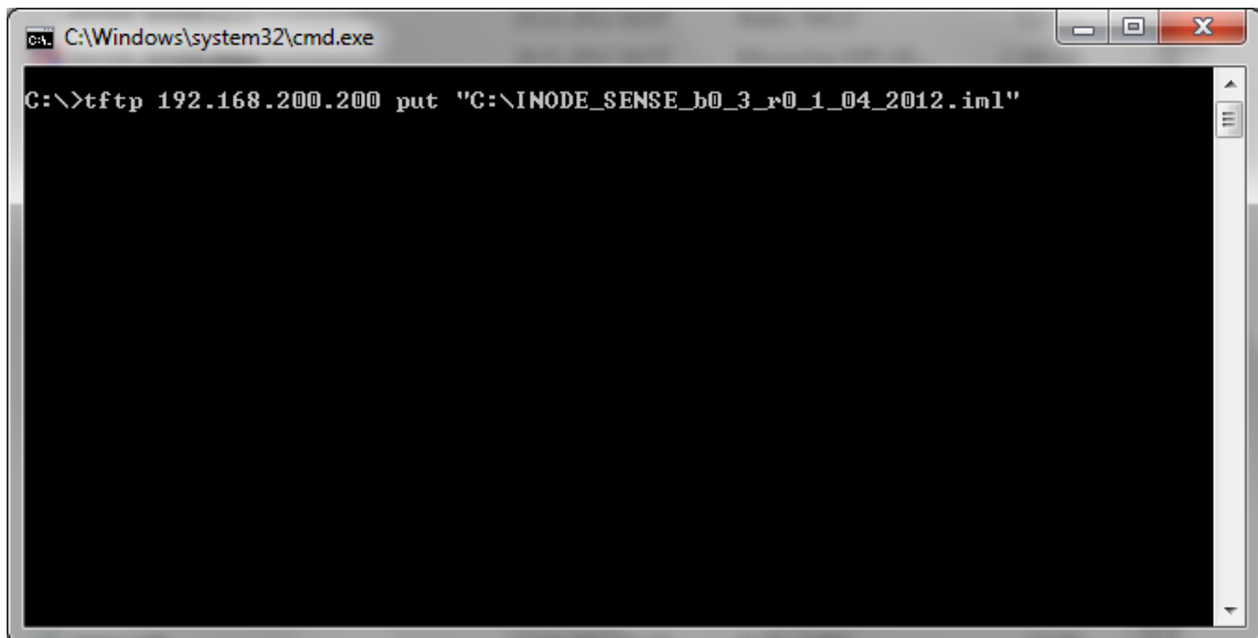
Рисунок 22 – Пример команды tftp для обновления ПО микроконтроллера iNode
