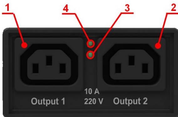
Рисунок 2 – Внешний вид задней панели устройства
