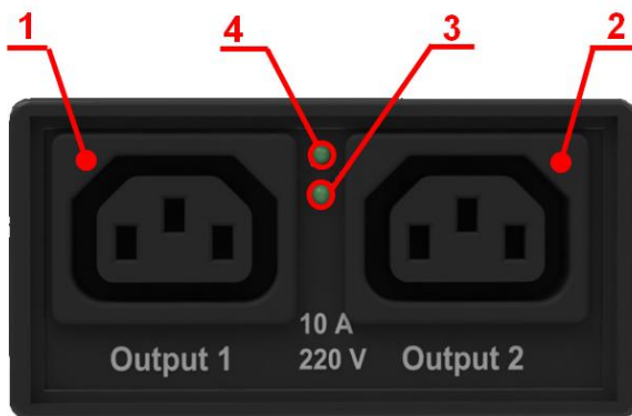
Рисунок 2 – Внешний вид передней панели устройства
