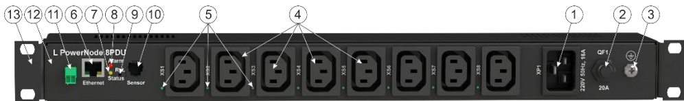
Рисунок 1 – Внешний вид и назначение органов управления и индикации LPowerNode 8PDU
