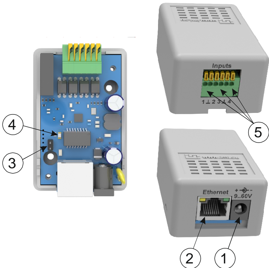
Рисунок 1 – Внешний вид передней панели адаптера iNode-Mini-D
