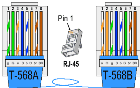
Рисунок 2 – Схема электрическая сетевого кабеля Ethernet 100Base-TX
