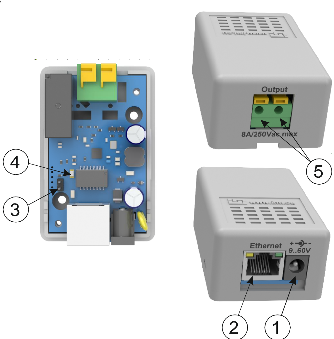
Рисунок 1 – Внешний вид адаптера iNode-Mini-R
