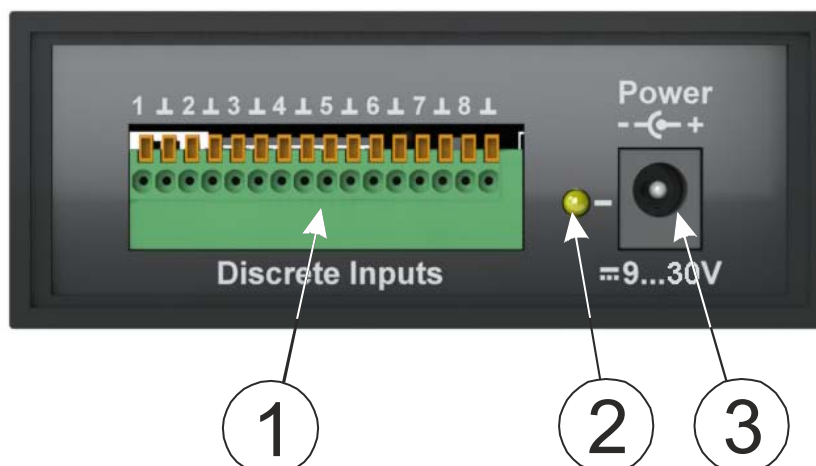
Рисунок 2 – Внешний вид задней панели адаптера iNode-Sense
