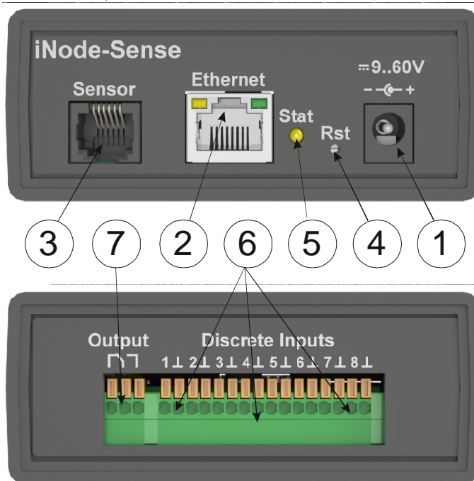
Рисунок 1 – Внешний вид адаптера iNode-Sense
